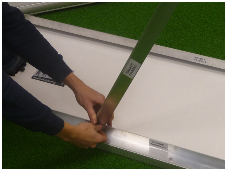
Etape 2 : Bras de liaison
