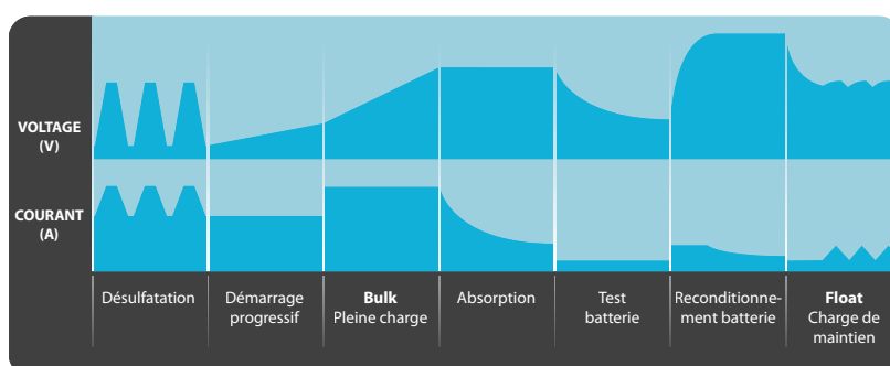
Courbe de charge
